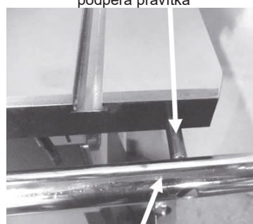
vymezovač pravítka
